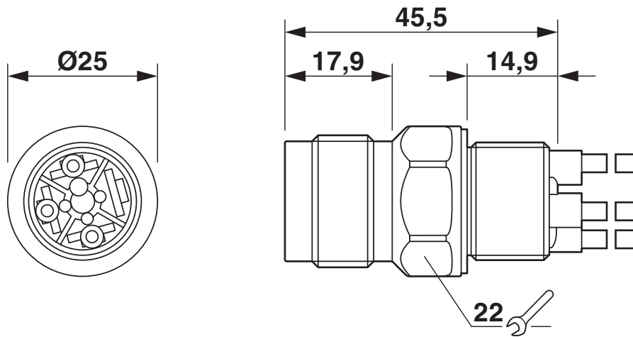
Rysunek wymiarowy
