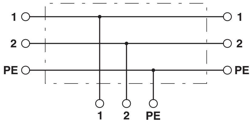
Schemat
