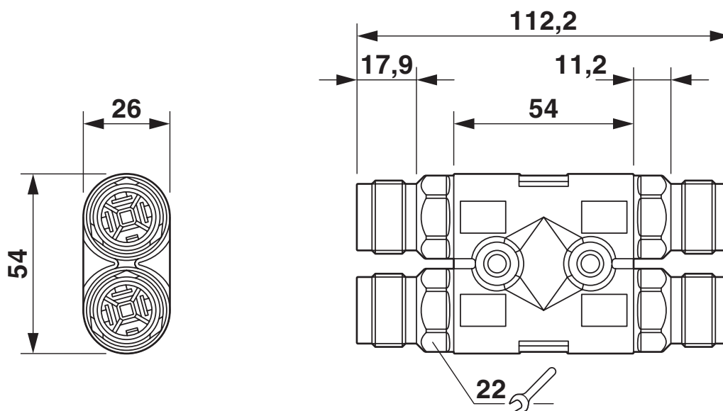
Rysunek wymiarowy
