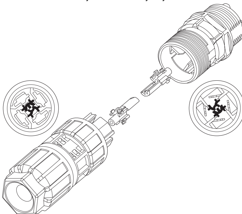
Rysunek schematyczny
