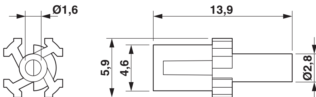
Rysunek wymiarowy
