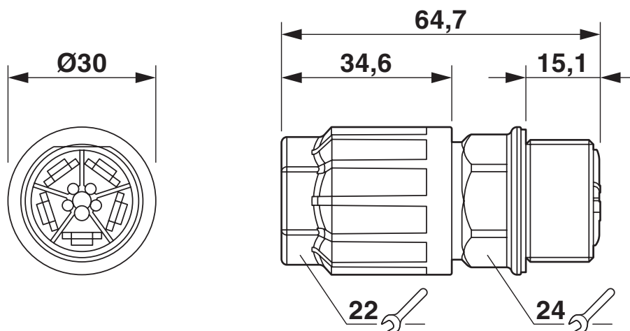
Rysunek wymiarowy
