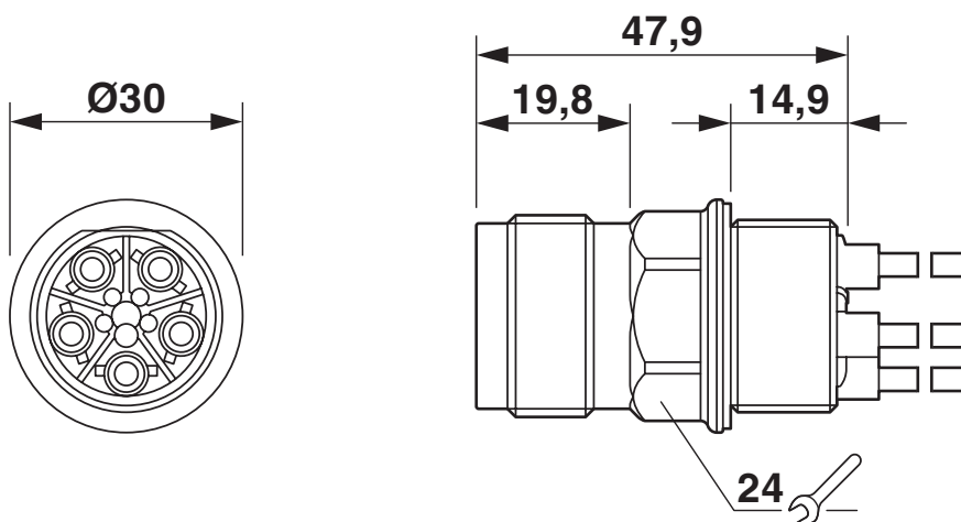
Rysunek wymiarowy
