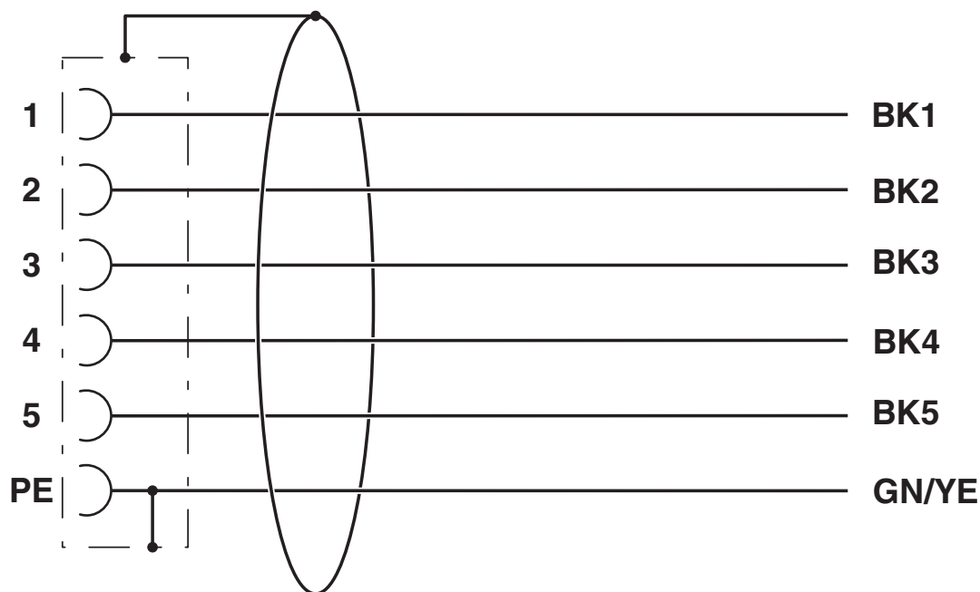
Schemat
