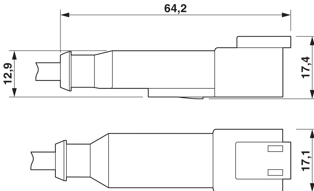
DEUTSCH DT04-2P, widok z góry i widok z boku
