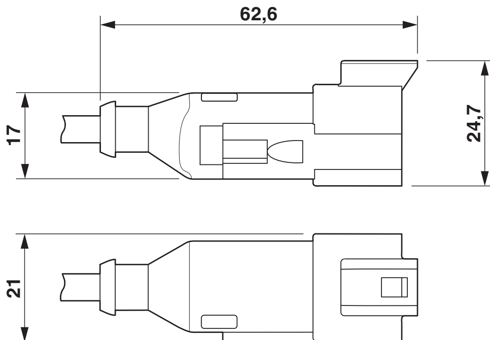
DEUTSCH DT04-3P, widok z góry i widok z boku
