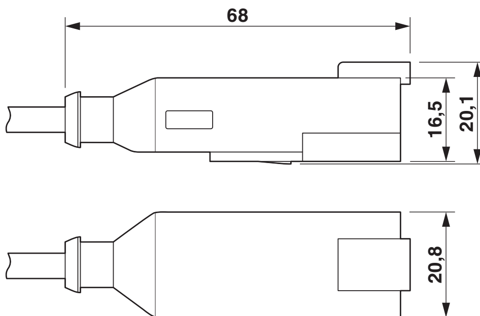
Rysunek wymiarowy
