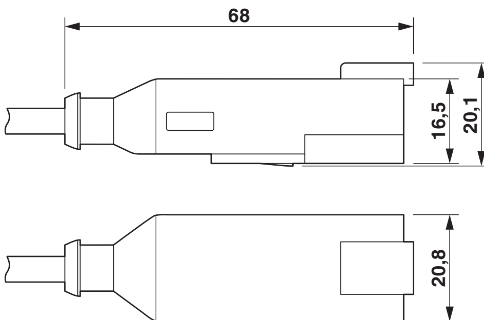
Rysunek wymiarowy
