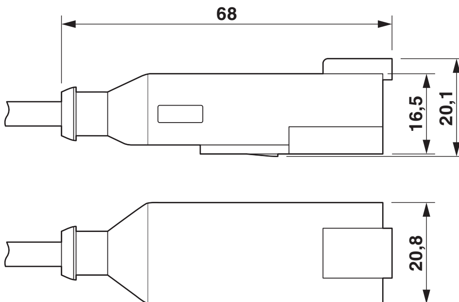
DEUTSCH DT04-4P, widok z góry i widok z boku
