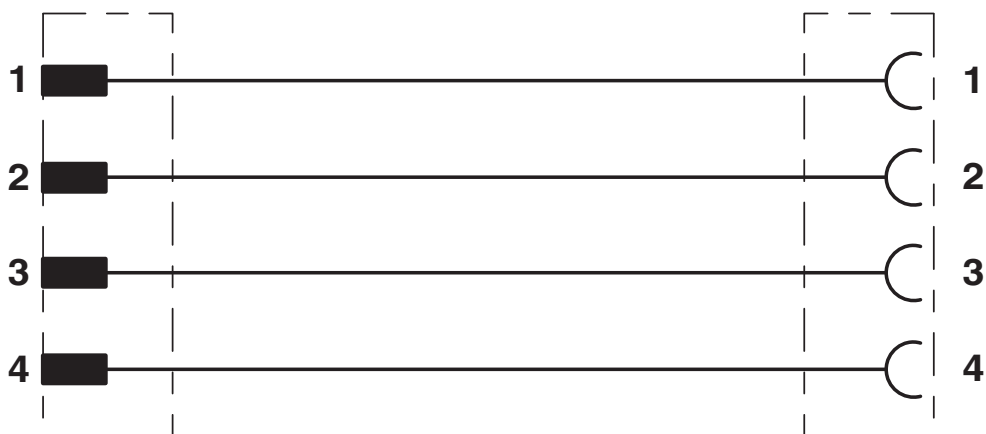
Schemat
