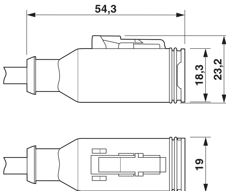
Rysunek wymiarowy
