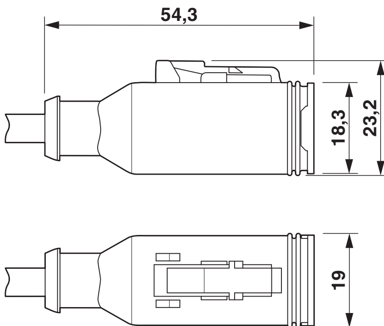
DEUTSCH DT06-3S, widok z góry i widok z boku
