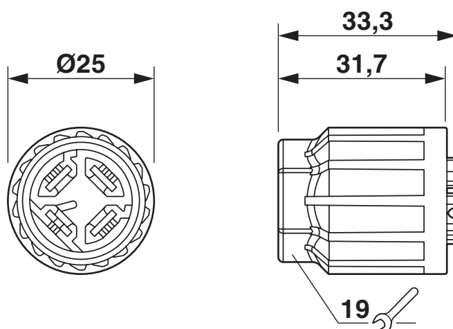
Rysunek wymiarowy
