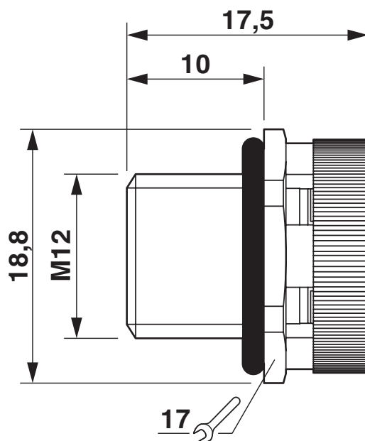
Rysunek wymiarowy
