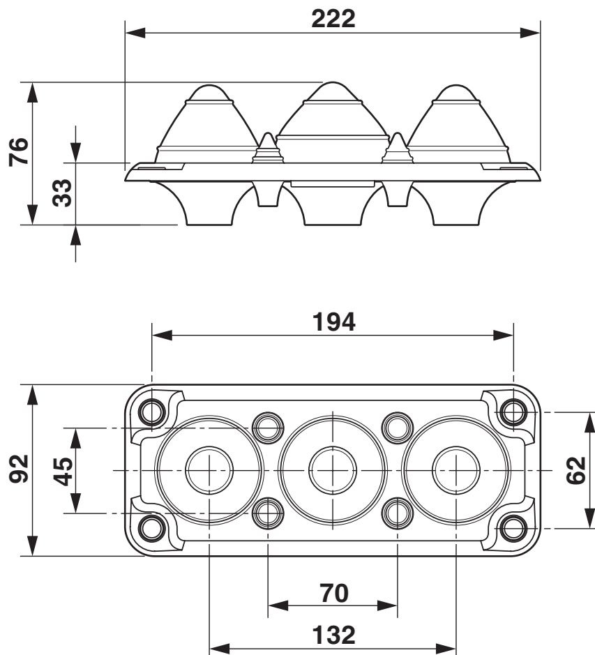
Rysunek wymiarowy
