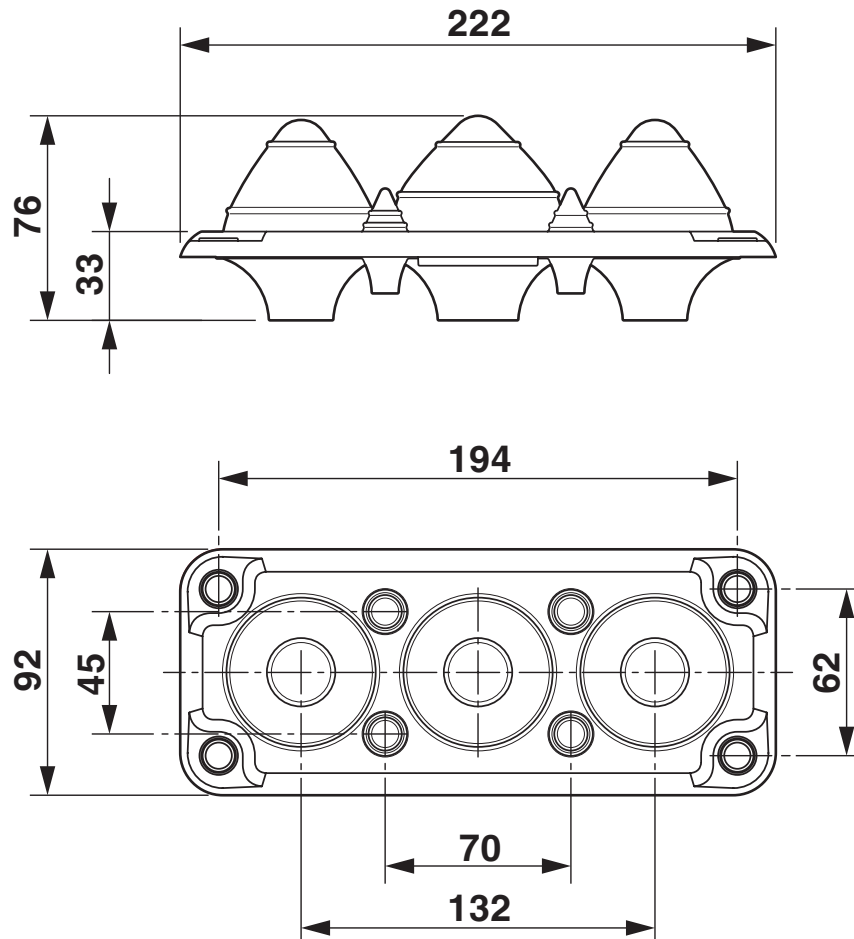
Rysunek wymiarowy
