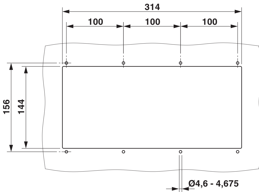
Rysunek otworów w ścianie
