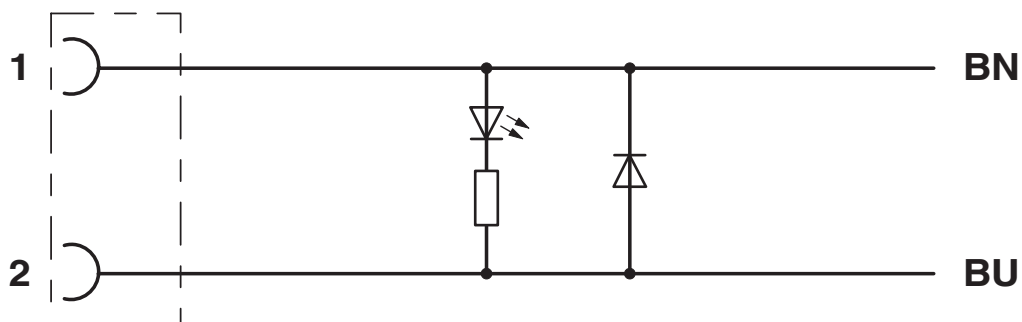
Schemat
