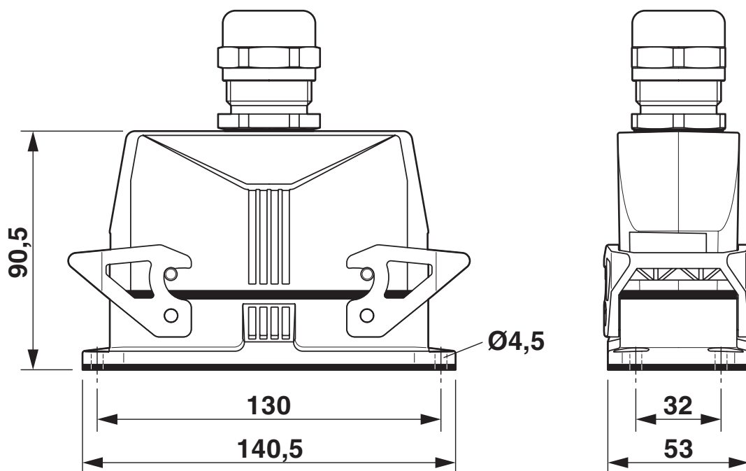
Rysunek wymiarowy
