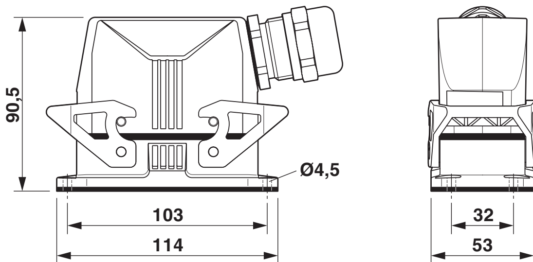
Rysunek wymiarowy
