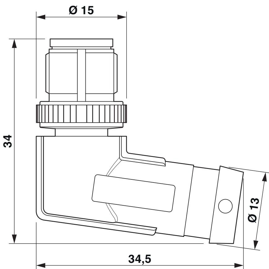
Rysunek wymiarowy
