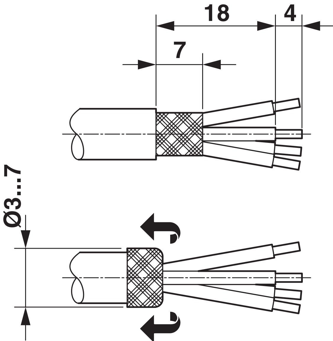
Rysunek wymiarowy
