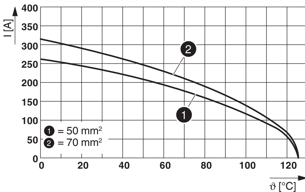
Dwa moduły w obudowie B24
