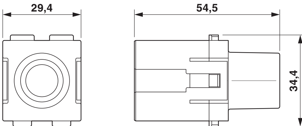
Rysunek wymiarowy
