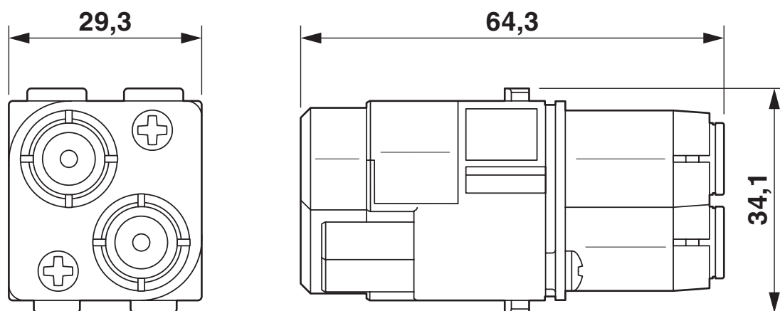
Rysunek wymiarowy
