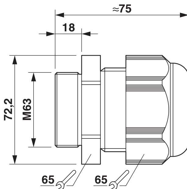
Rysunek wymiarowy
