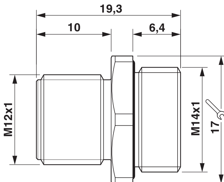
Rysunek wymiarowy
