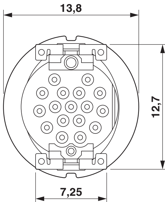
Rysunek wymiarowy
