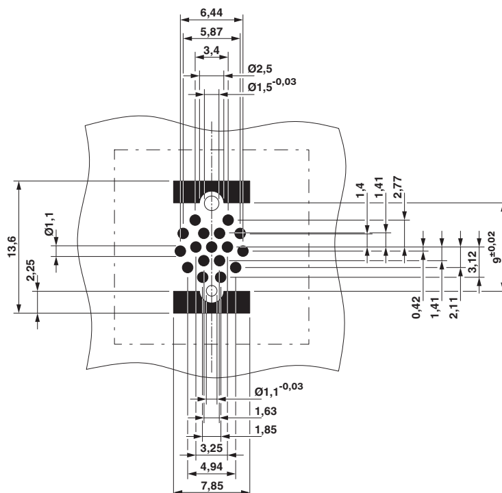
Otworowanie/geometria płytek lutowniczych
