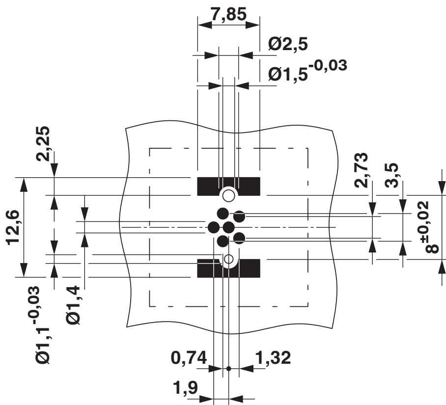
Rysunek wymiarowy
