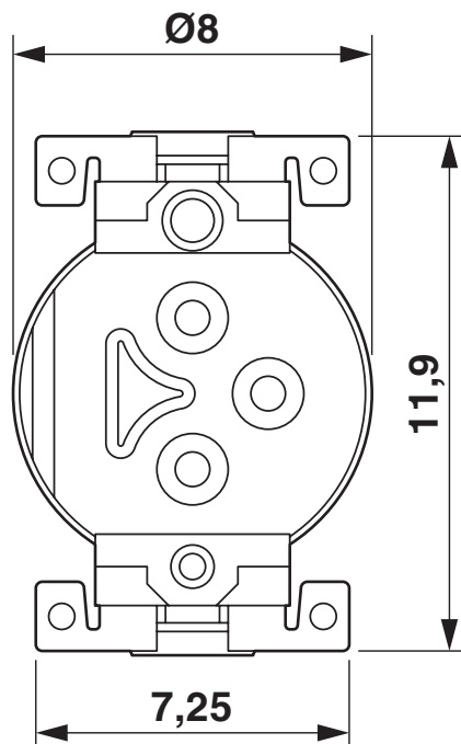
Rysunek wymiarowy
