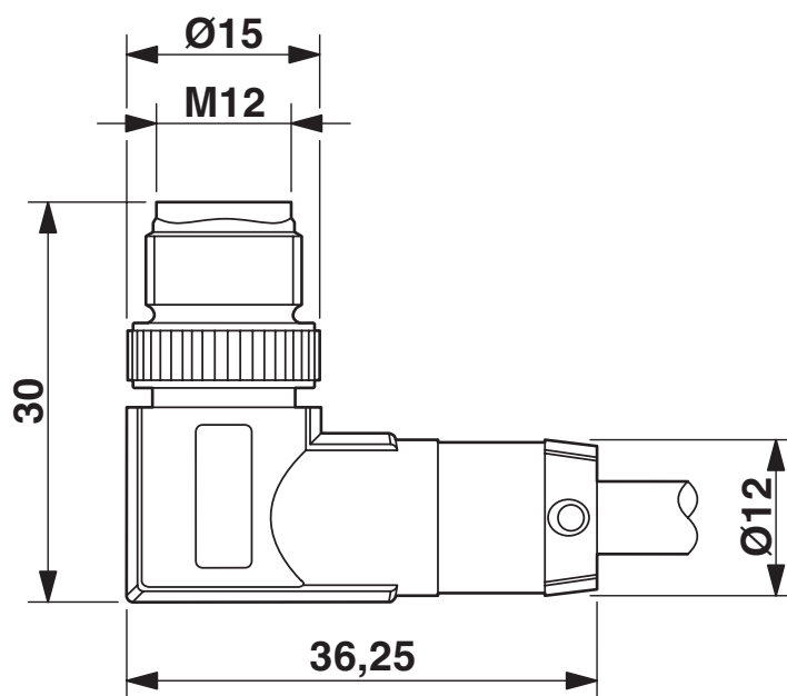
Rysunek wymiarowy
