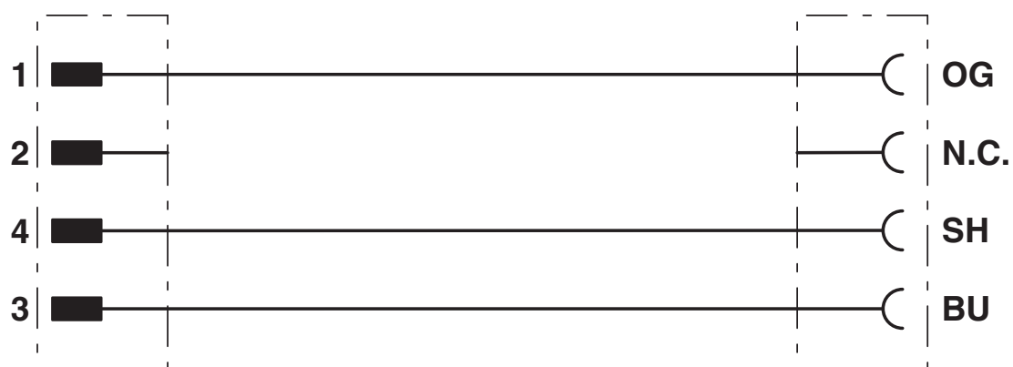
Schemat
