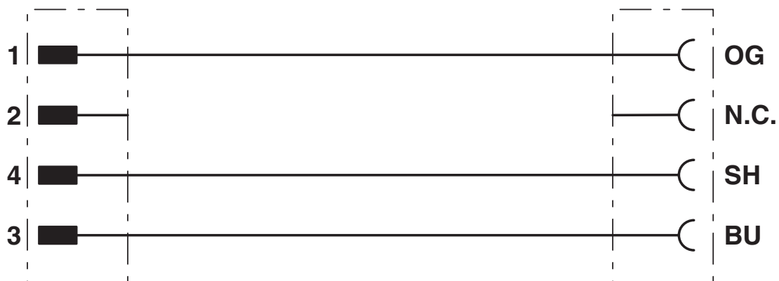
Schemat
