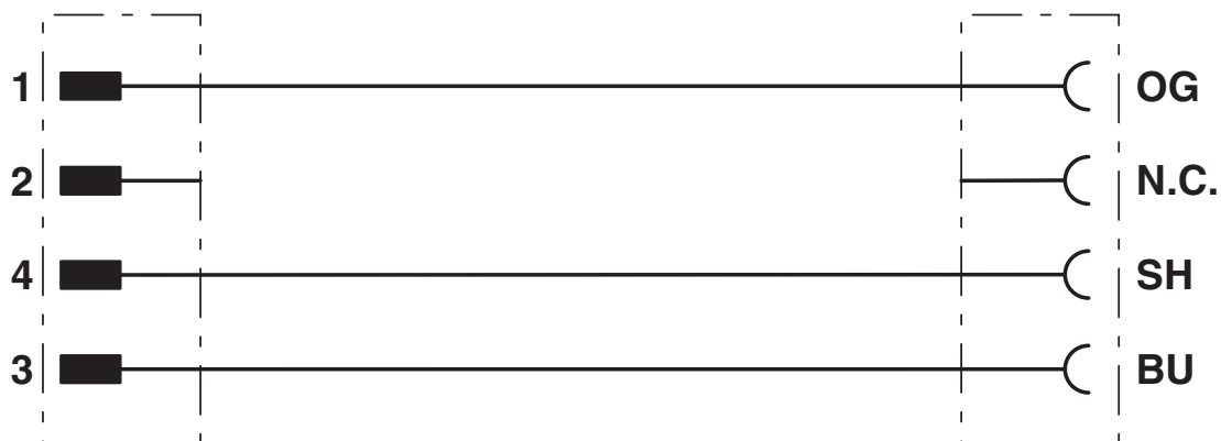
Schemat
