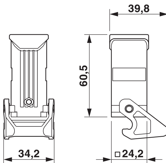
Rysunek wymiarowy
