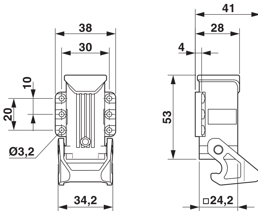
Rysunek wymiarowy
