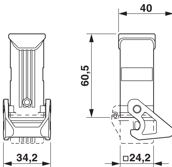
Rysunek wymiarowy
