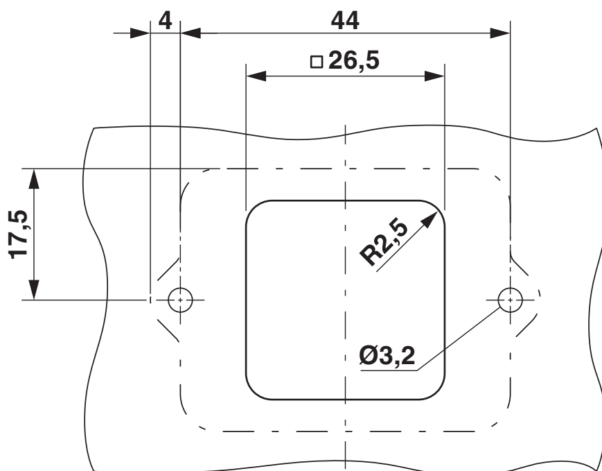
Rysunek wymiarowy
