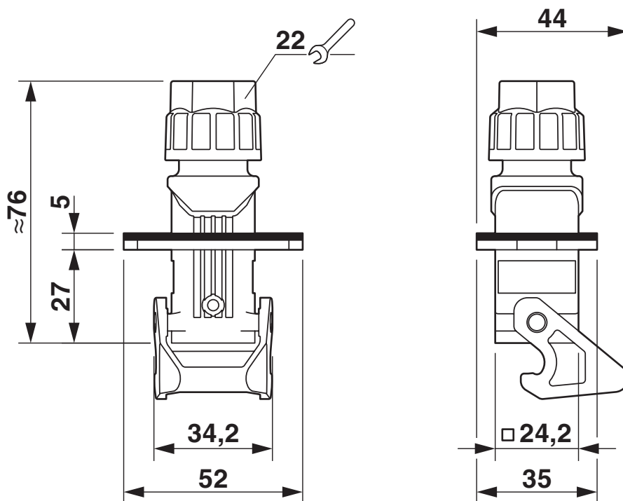
Rysunek wymiarowy
