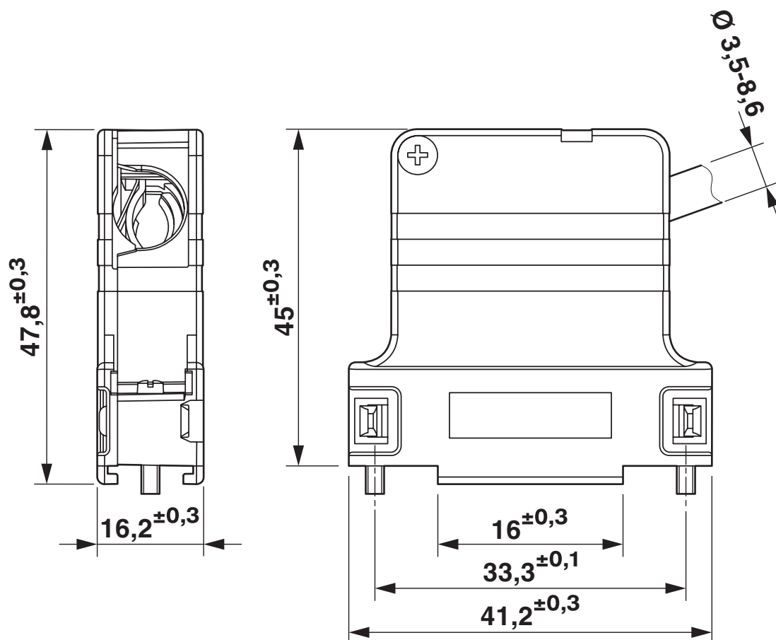
Rysunek wymiarowy
