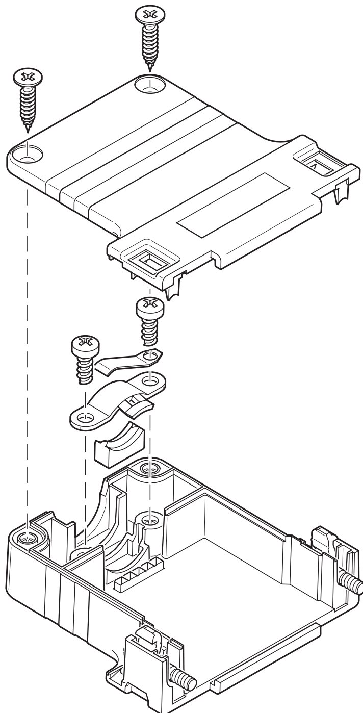
Rysunek schematyczny
