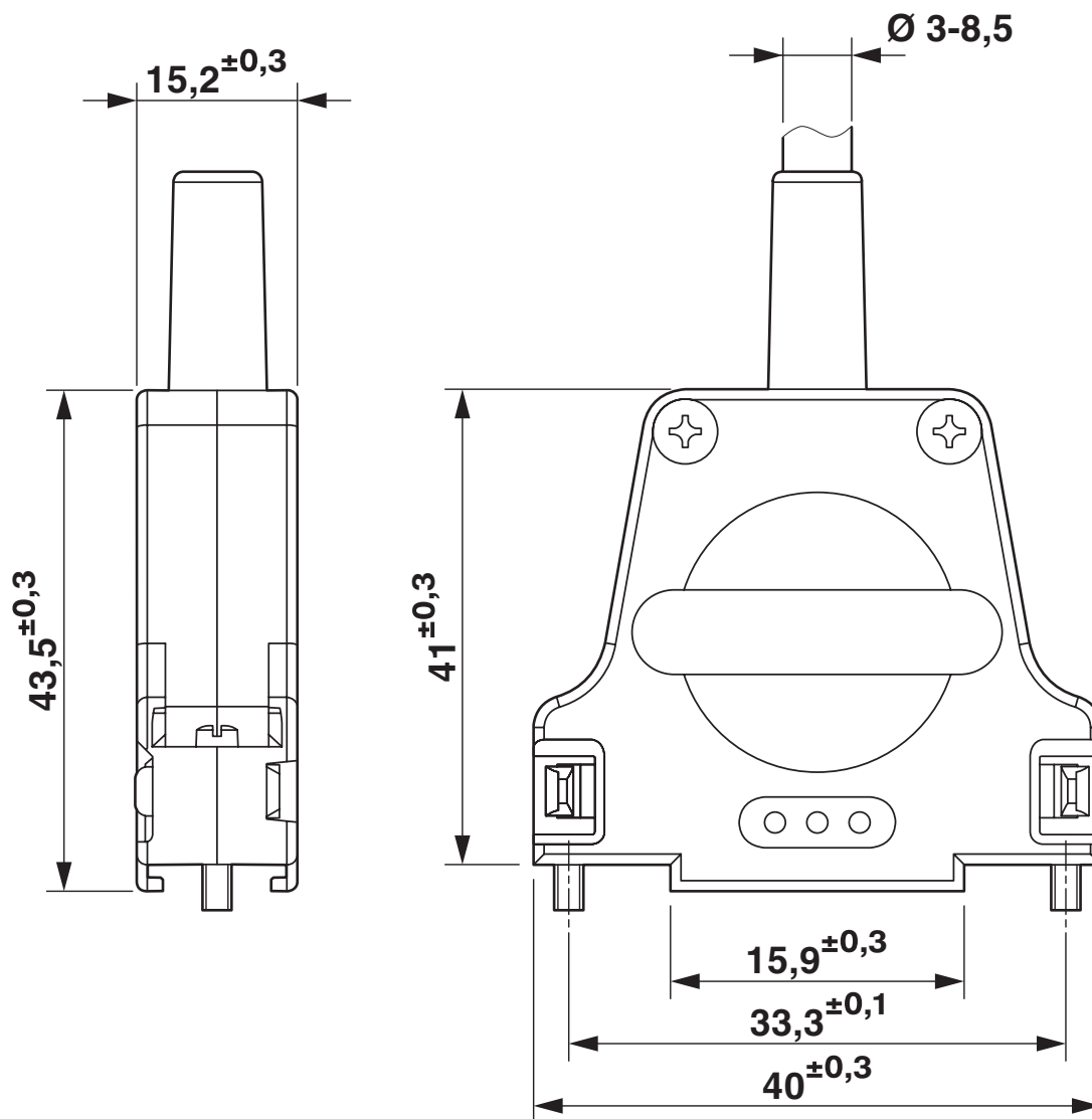
Rysunek wymiarowy
