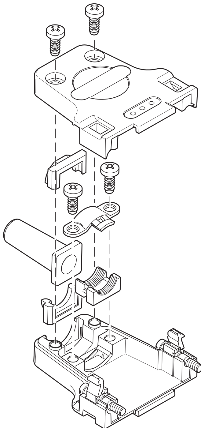
Rysunek schematyczny
