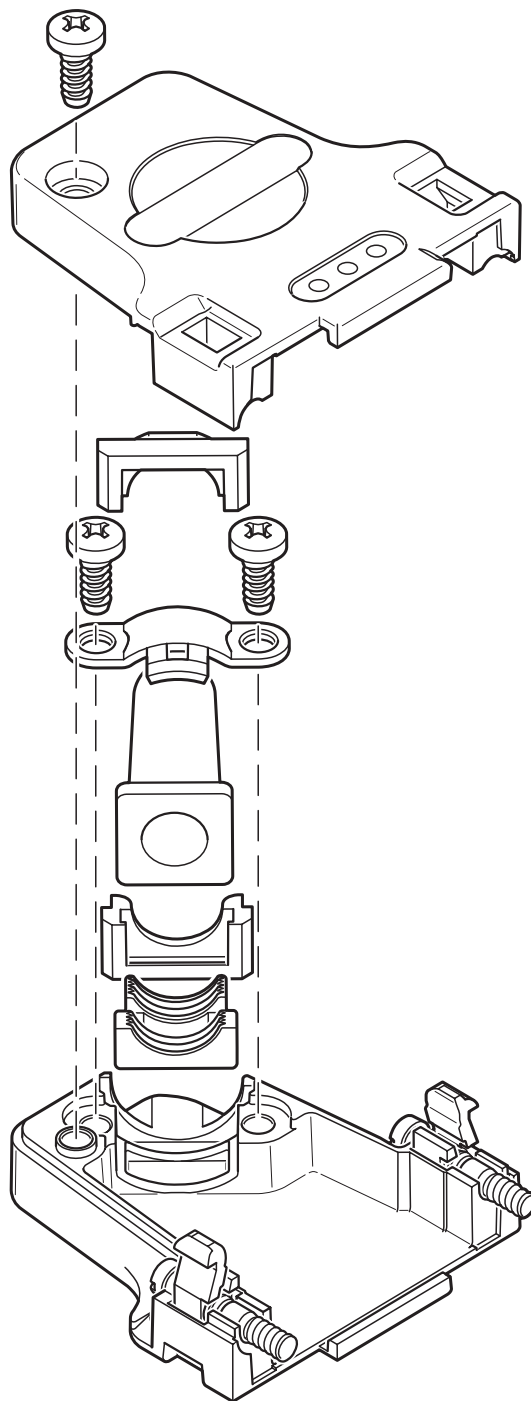
Rysunek schematyczny
