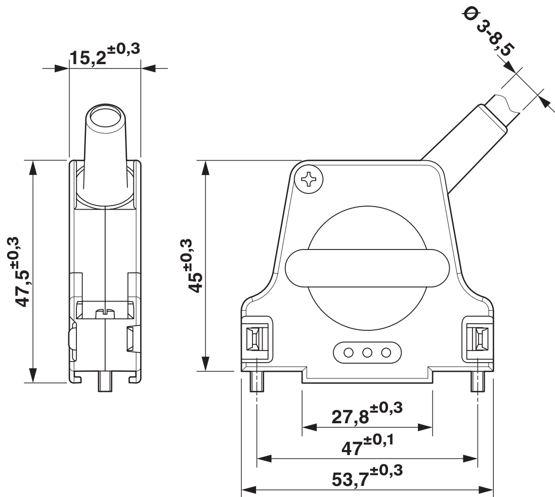
Rysunek wymiarowy
