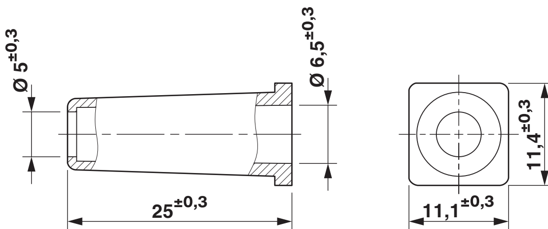
Rysunek wymiarowy
