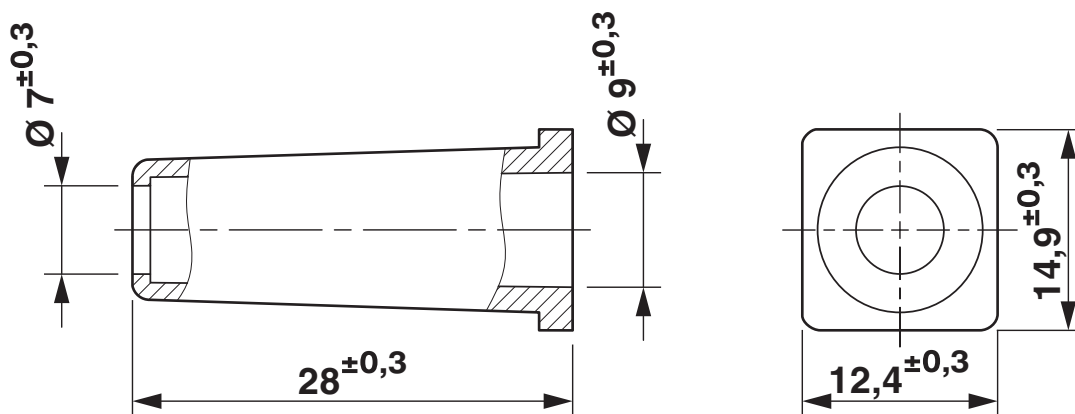
Rysunek wymiarowy
