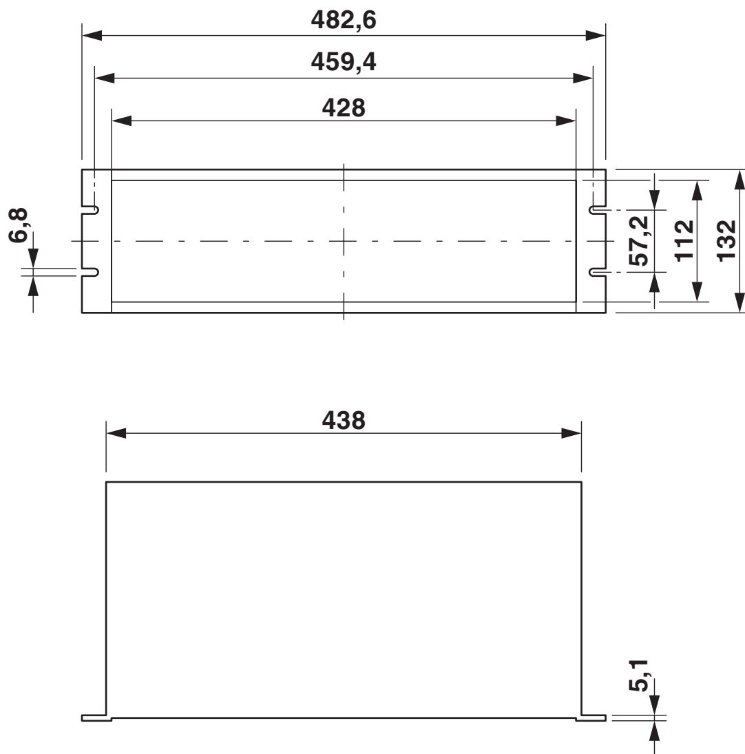
Rysunek wymiarowy
