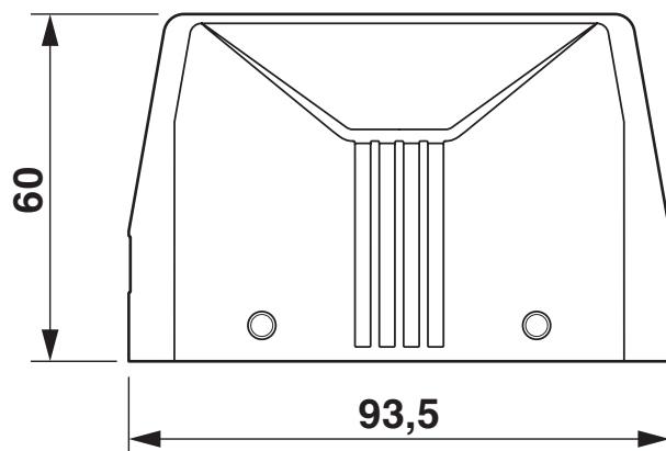
Rysunek wymiarowy
