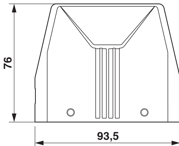
Rysunek wymiarowy
